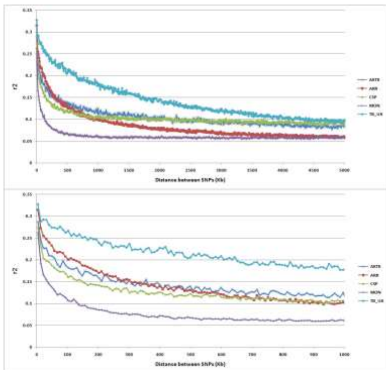
شکل ۲. نقشه فرسایش LD محاسبه شده به روش r^2 بین جفت SNPهای مجاور در مقابل فاصله نشانگری در تمام کروموزومها. شکل بالا: فاصله نشانگری در دامنه ۵۰۰۰-۰ Kb، شکل پایین: فاصله نشانگری در دامنه ۱۰۰۰-۰ Kb. Figure 2. LD decay map measured by r^2 between SNP pairs according to distance with all chromosomes. Upper: Distance range from 0 to 5000 Kb. Lower: Distance range from 0 upto 1000 kb. AKTK: AkhalTake, ARR: Arrabian, CSP: Caspian, MON: Mongolian, TB_UK: Thoroughbered horses breeds.
