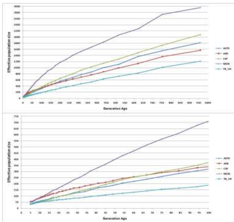
شکل ۳. روند تغییر اندازه مؤثر جمعیت ( N_e ) در طی نسل‌های گذشته. شکل بالا: فاصله بین ۱۰۰۰-۵ نسل، شکل پایین: فاصله بین ۱۰۰-۵ نسل گذشته. Figure 3. Effective population size ( N_e ) trend plotted against generations in the past, truncated at Upper: Distance range from 5 to 1000 generations. Lower: Distance range from 5 upto 100 generations ago. AKTK: AkhalTake, ARR: Arrabian, CSP: Caspian, MON: Mongolian, TB_UK: Thoroughbered horses breeds.
