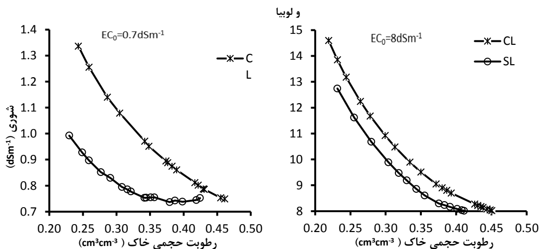
شکل ۴. تغییرات شوری خاک به صورت تابعی از رطوبت خاک لوم شنی (SL) و لوم رسی (CL)، تحت شوری‌های اولیه (EC 0 ) ۷/۱ و ۸ دسی زیمنس بر متر
