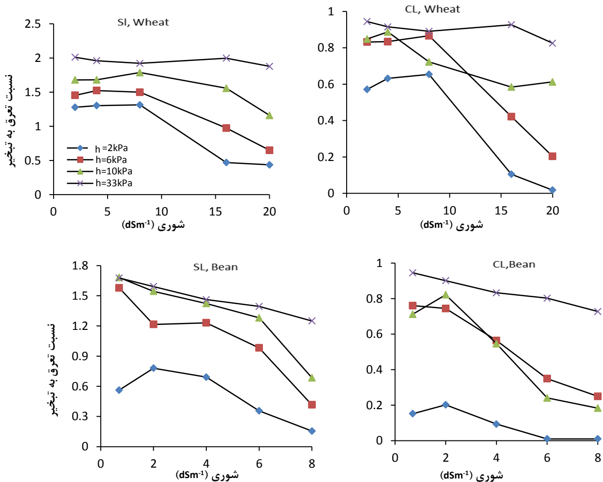
شکل ۳. تغییرات میزان نسبت تعرق به تبخیر به صورت تابعی از شوری تحت مکش‌های ماتریک مختلف در خاک لوم شنی (SL) و لوم رسی (CL) برای گیاه گندم
