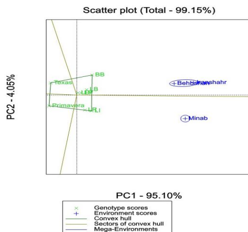
شکل ۵. نمودار چندضلعی GGE biplot برای گروه‌بندی محیط‌ها بر اساس درصد ماده خشک سوخ Figure 5. Polygonograph of GGE biplot method for grouping environments based on dry matter percentage. LP: Landrace Paddock, BB: Bred Behbahan, LBr: Landrace Brazjan, LI: Landrace Iranshahr, LR: Landrace Ramhormoz, Primavera: Primavera cultivar, Texas: Texas Early Grano cultivar, LB: Landrace Behbahan
