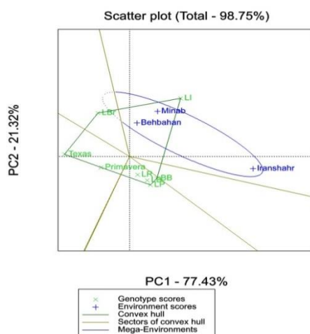
شکل ۱. نمودار چندضلعی GGE biplot برای گروه‌بندی محیط‌ها بر اساس بولتینگ
