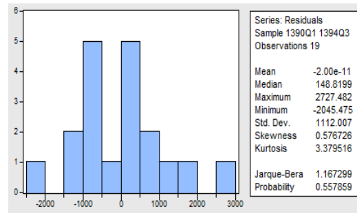
شکل ۷. آزمون نرمالیتی فروش
