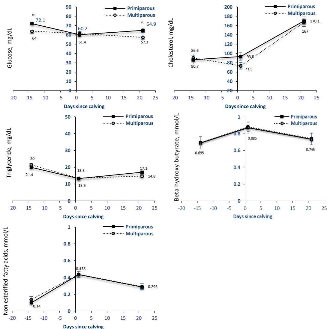
شکل ۲. متابولیت‌های شاخص انرژی خون گاوهای یک و چندبار زایش طی دوره انتقال.
