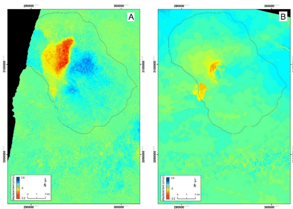
شکل ۱۰. نقشه جابه‌جایی مقطعی، A: بین تاریخ ۲۰۰۷/۳/۲۰-۲۰۰۷/۱۲/۱۵؛ B: بین تاریخ ۲۰۰۷/۱۱/۱۷-۲۰۰۸/۴/۸. همه تصاویر به صورت بالاگذردند
