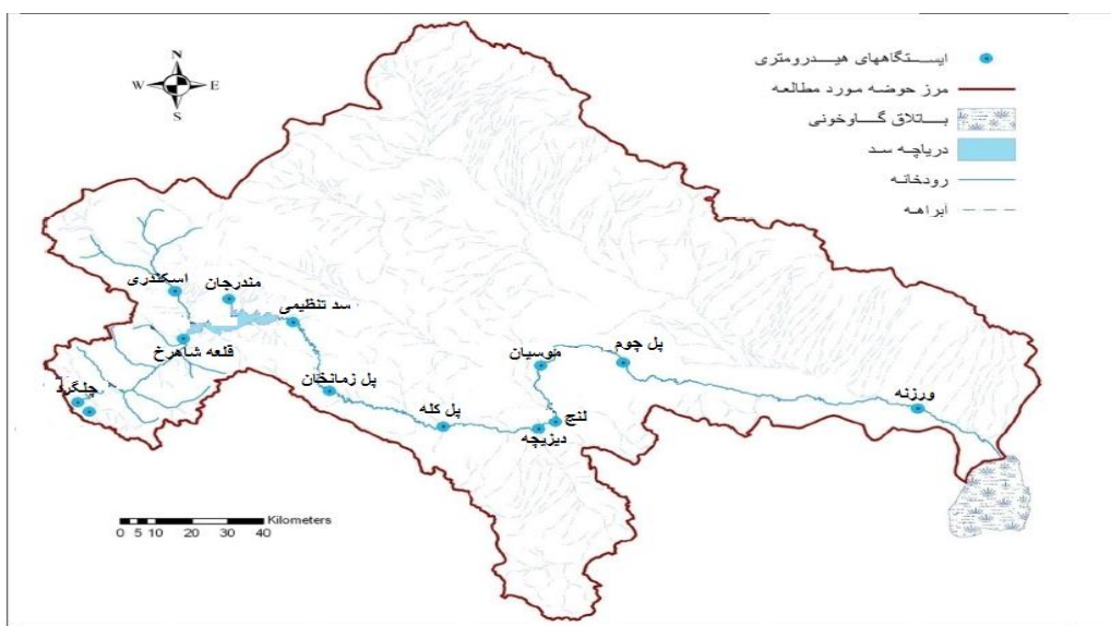
شکل ۱- نقشه موقعیت ایستگاههای هیدرومتری در رودخانه زاینده رود
