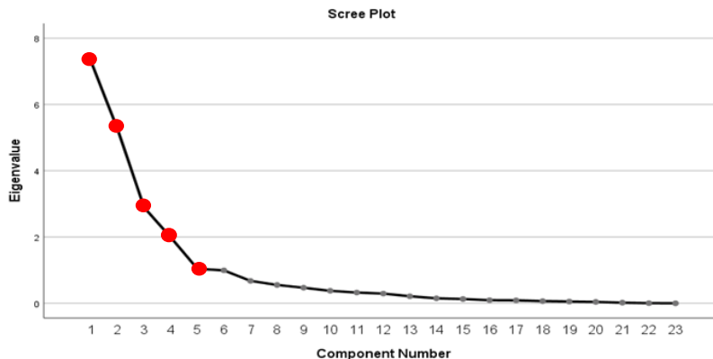
شکل ۵. نمودار تغییرات ارزش ویژه تجزیه مؤلفه‌های اصلی
