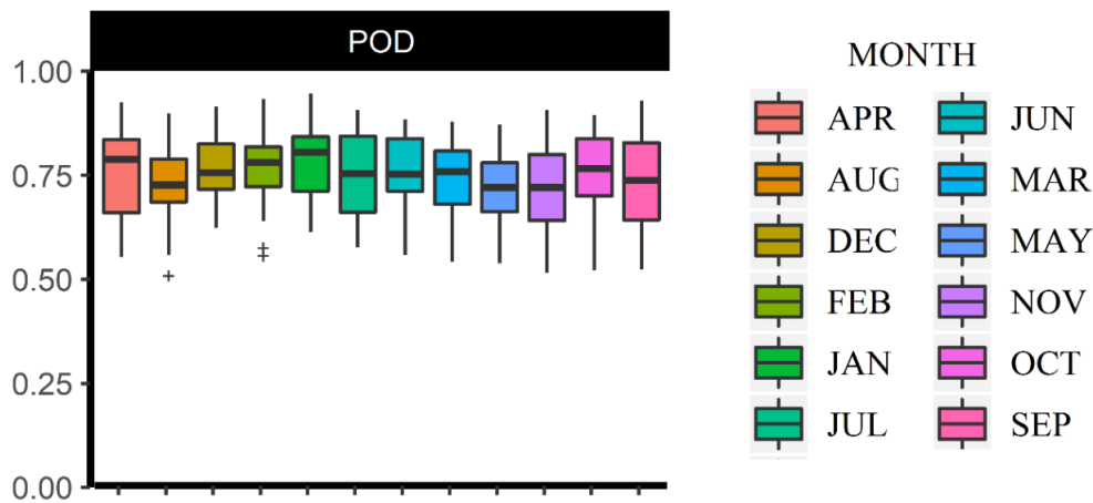
شکل ۱۰- جعبه‌ای شاخص POD جدول توافقی طی دوره آماری ۲۰۰۴ تا ۲۰۱۴
