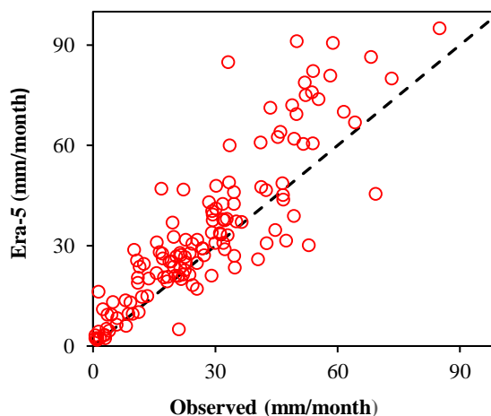
شکل ۳- عملکرد منبع بارشی Era5 در تخمین بارش میانگین روزانه و ماهانه کل ایستگاه‌های مطالعاتی در سطح استان اردبیل
