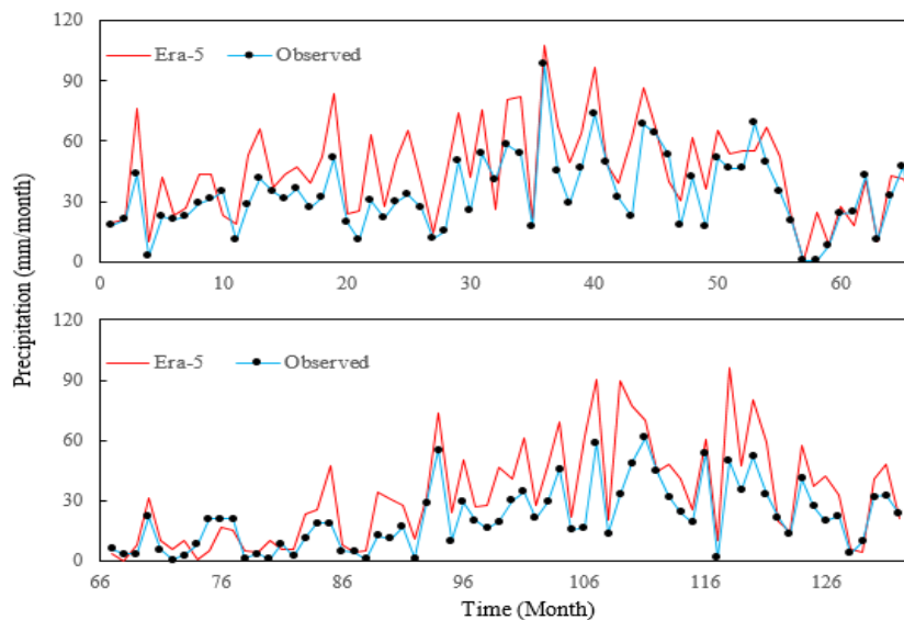
شکل ۴- سری زمانی بارش میانگین ایستگاه‌های زمینی و منبع بارش Era5 در مقیاس زمانی ماهانه
