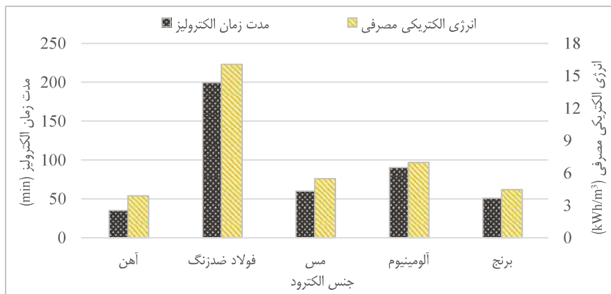
شکل ۱. نتایج مقایسه جنس الکتروودهای مورد استفاده در سامانه بر اساس مدت زمان الکترولیز و انرژی الکتریکی مصرفی
