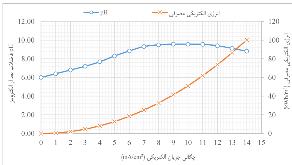
شکل ۳. نتایج بررسی تغییرات pH فاضلاب بعد از الکترولیز و انرژی الکتريکى مصرفی سامانه برحسب چگالی جریان الکتريکى
