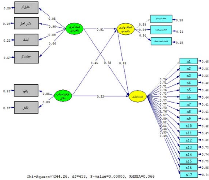
شکل ۱. مدل ساختاری متغیرهای تحقیق در حالت استاندارد
