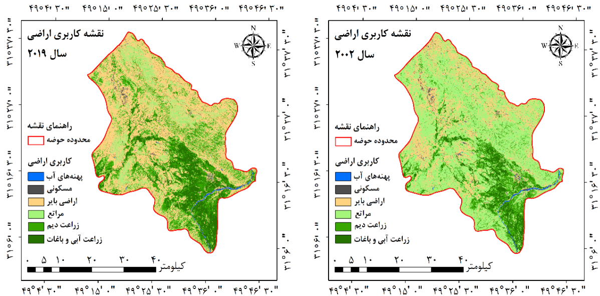
شکل ۳- نقشه‌های کاربری اراضی سال‌های ۲۰۱۹ و ۲۰۰۲
