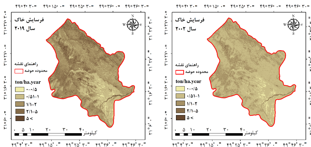
شکل ۵- نقشه‌های فرسایش خاک برای سال‌های ۲۰۱۹ و ۲۰۰۲
