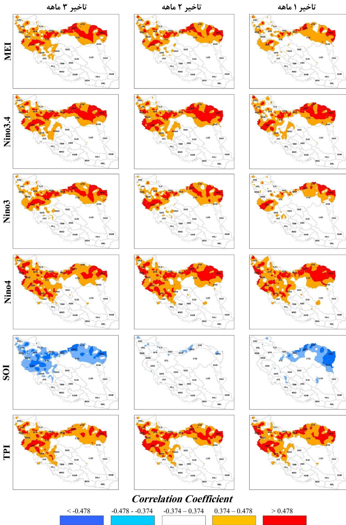
شکل ۵- پراکنش ضریب همبستگی شاخص‌های مرتبط با ENSO و TPI با تاخیر ۳ تا ۱ ماه (ژانویه تا مارس)
