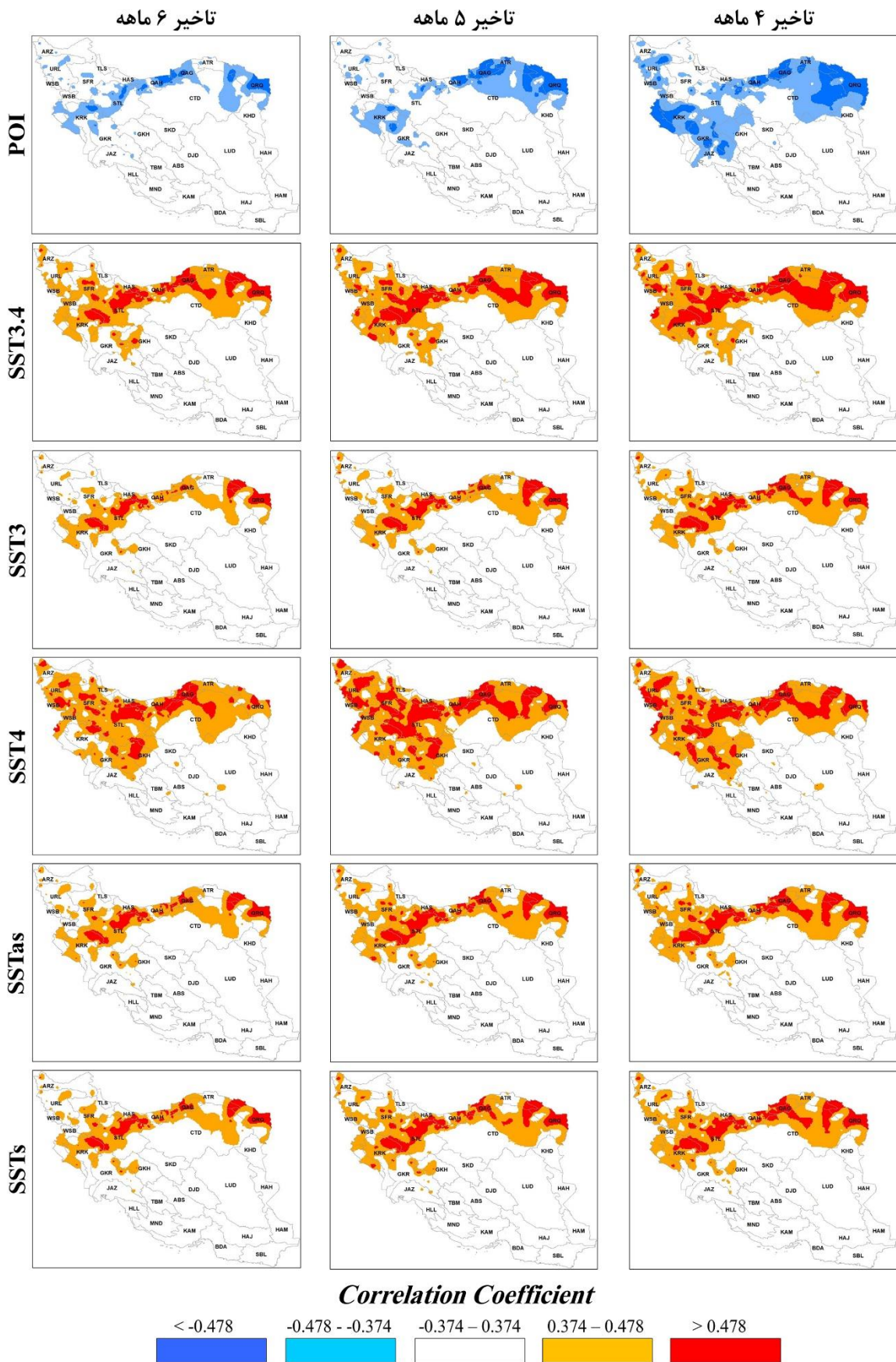
شکل ۶- پراکنش ضریب همبستگی شاخص‌های مرتبط با SST ها و POI با تاخیر ۴ تا ۶ ماه (اکتبر تا دسامبر)
