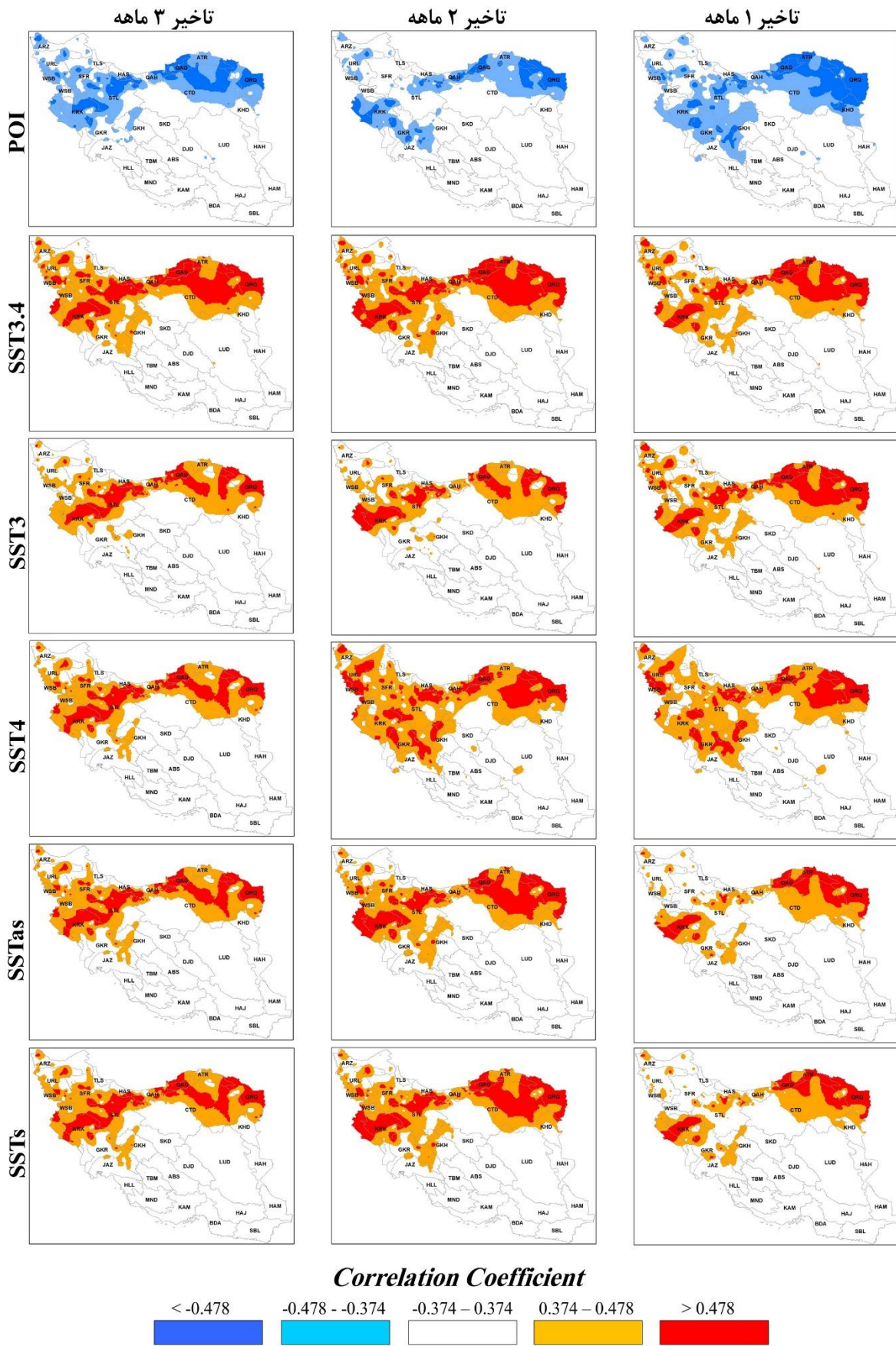
شکل ۷- پراکنش ضریب همبستگی شاخص‌های مرتبط با SST ها و POI با تاخیر ۱ تا ۳ ماه (ژانویه تا مارس)
