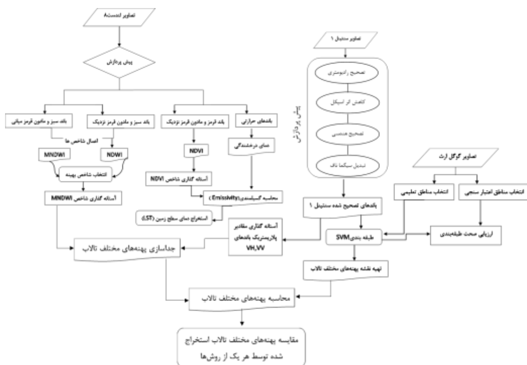
شکل ۲. فلوچارت تحقیق
