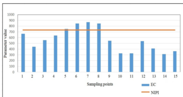
b- NIPI and EC values
