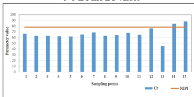
d- NIPI and Cr values
