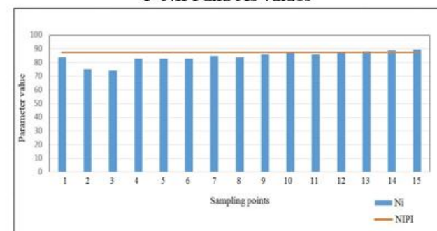
h- NIPI and Ni values
