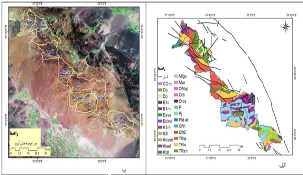
شکل شماره ۱. الف) نقشه‌ی گسل و زمین‌شناسی حوضه‌های آبریز جنوب ارتفاعات کرکس؛ ب) تصویر ماهواره‌ای حوضه‌های آبریز جنوب ارتفاعات کرکس
