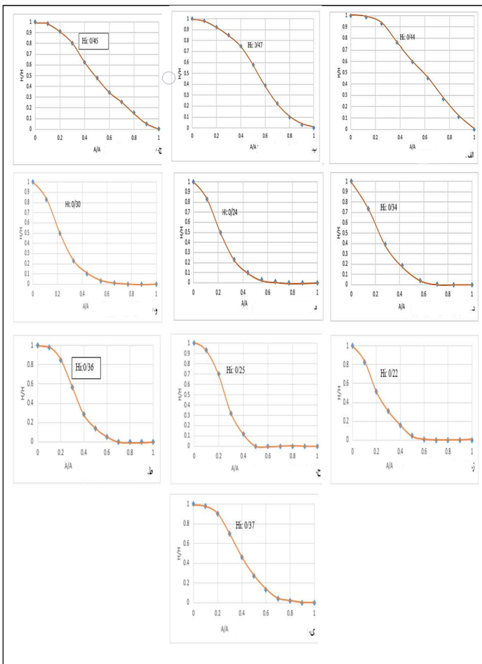
شکل شماره ۵. منحنی‌های فرازنامی حوضه‌های آبریز منطقه مطالعاتی: الف) مراوند؛ ب) نیازمرغ؛ ج) سه؛ د) کلهرود؛ م) آسنجد؛ و) رباط؛ ز) صفی‌آباد؛ ح) مرغ؛ ط) پناوند؛ ی) حبیب‌آباد
