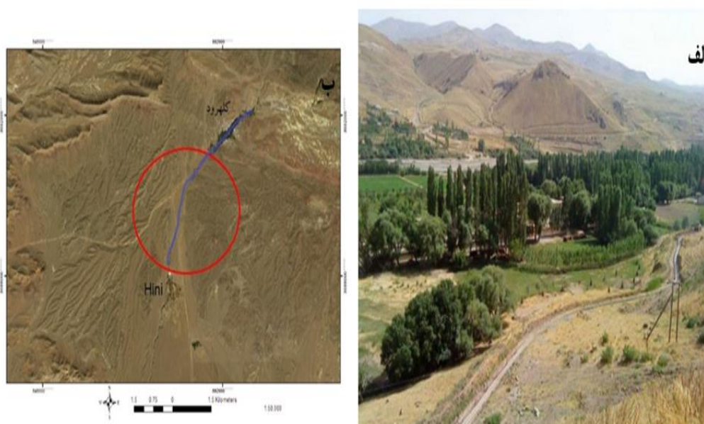
شکل شماره ۷. الف) دره رودخانه کلهرود؛ ب) تغییر مسیر رودخانه کلهرود
