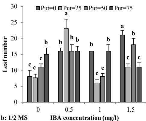
شکل ۴. مقایسه میانگین اثر متقابل ایندول بوتیریک اسید و پوتریسین بر تعداد برگ ریزنمونه‌های گل‌بای پایه پیروودوارف در محیط‌های کشت MS (A) و ۱/۲ MS (B). Figure 4. Mean comparison interaction effect of indole butyric acid and putrescine on leaf number of pyrodwarf rootstock explants in MS (A) and 1/2 MS (B) mediums.
