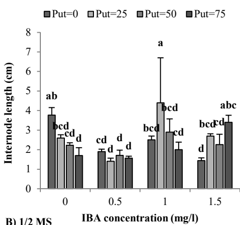
شکل ۶. مقایسه میانگین اثر متقابل ایندول بوتیریک اسید و پوتریسین بر طول میانگره ریزنمونه‌های گلابی پایه پیروودوارف در محیط کشت MS (A) و 1/2 MS (B).
