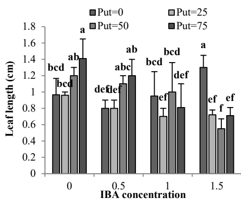
شکل ۵. مقایسه میانگین اثر متقابل ایندول بوتیریک اسید و پوتریسین بر طول برگ‌های باززایی شده ریزنمونه‌های گل‌بای پایه پیروودوارف در محیط کشت MS.
