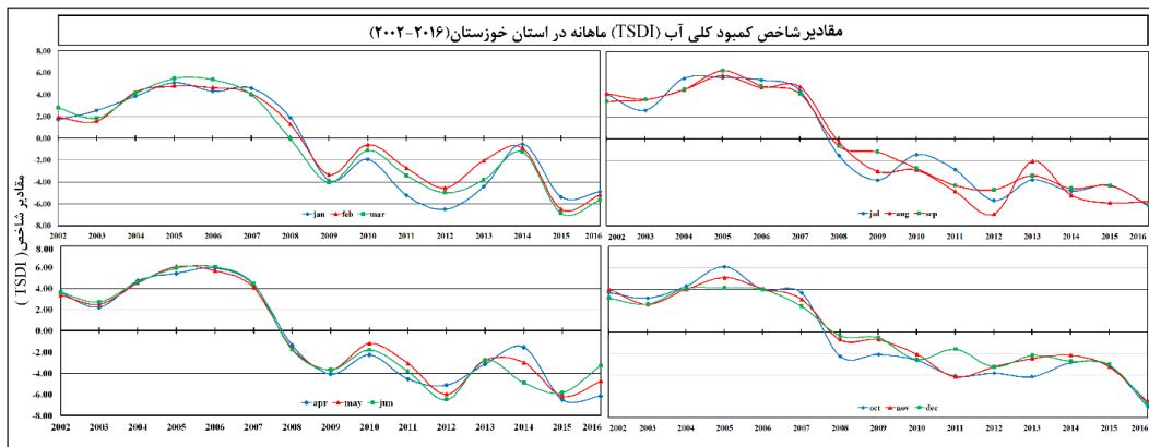
شکل ۶. مقادیر TSDI ماهانه در بازه ۲۰۰۲ تا ۲۰۱۶
