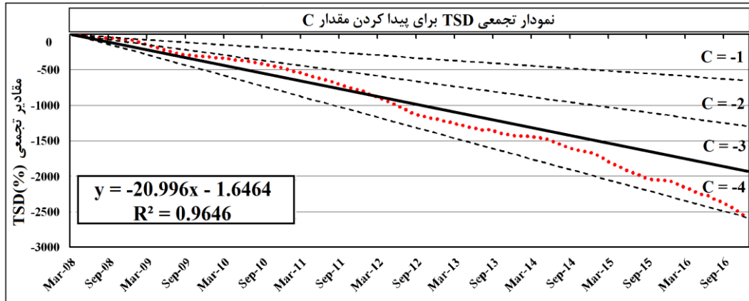
شکل ۵. نمودار تجمعی TSD و تقسیم فضا به ۴ قسمت مساوی
