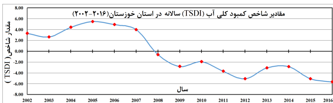
شکل ۸. مقادیر شاخص کلی آب TSDI سالانه در استان خوزستان (۲۰۰۲-۲۰۱۶)
