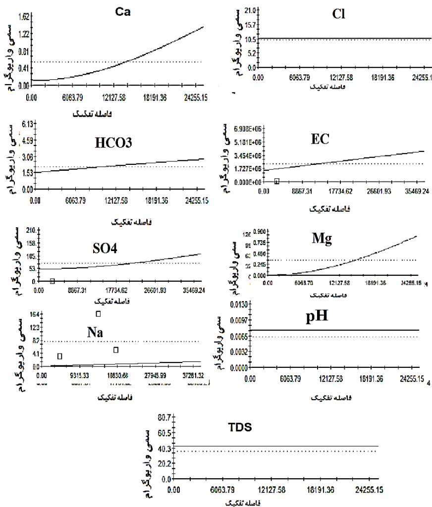
شکل ۷. نمودار واریوگرم متغیرهای کیفی منابع آب قنات
