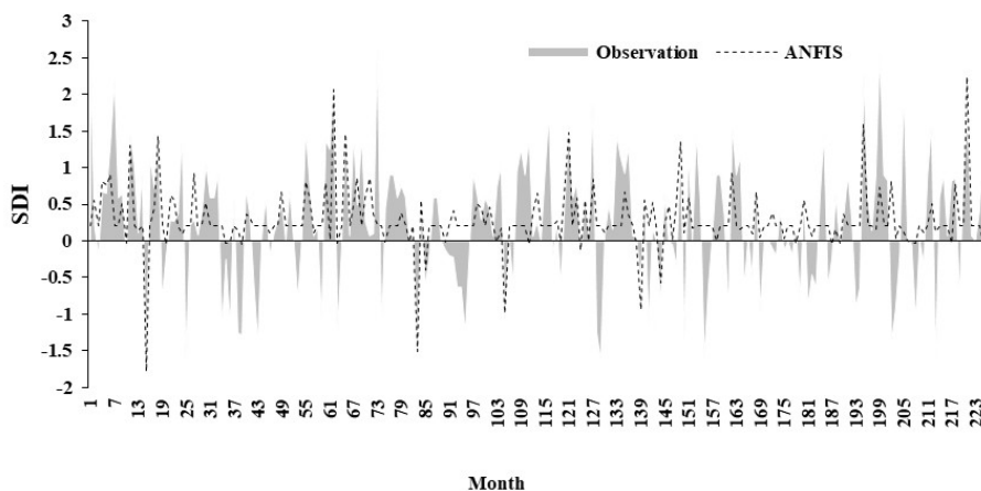
شکل ۶. نمودار سری زمانی داده‌های مشاهده‌شده شاخص SDI و شبیه‌سازی‌شده با استفاده از مدل‌های ANFIS و LS-SVR
