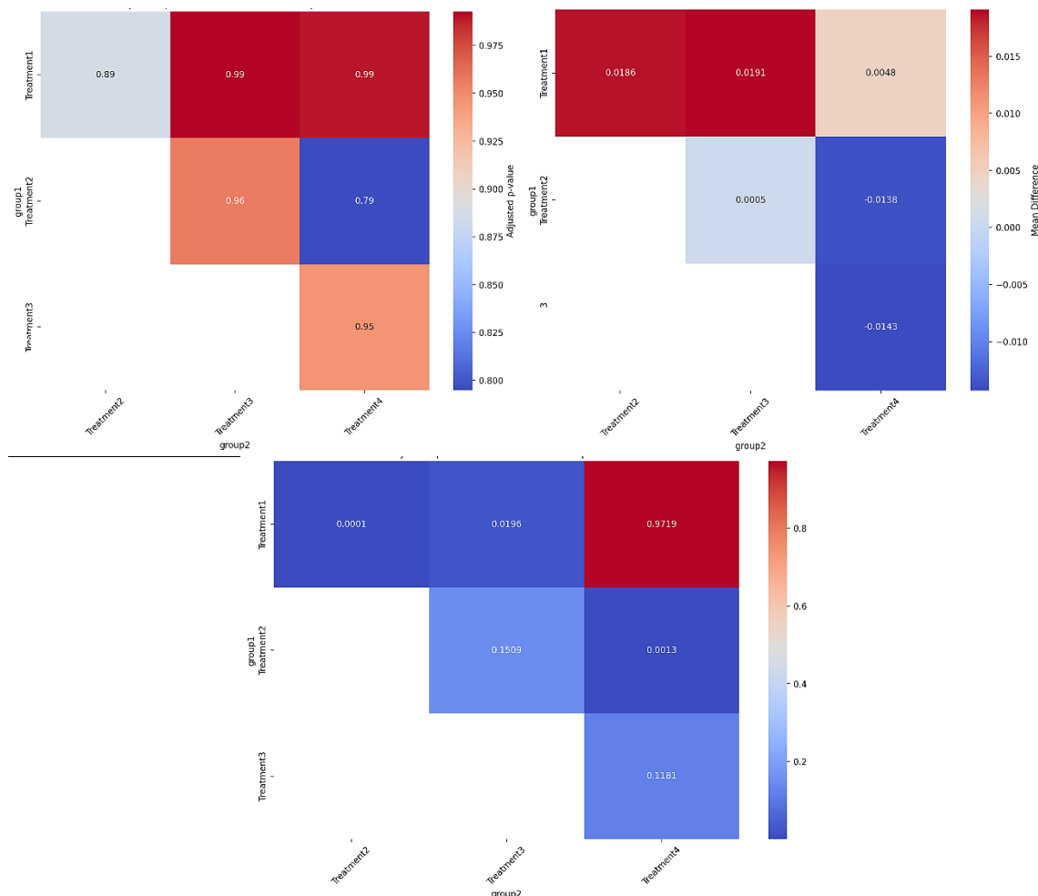
شکل ۷. نتایج آزمون تفاوت معناداری بین میانگین تیمارها الف) RMSE (ب) RRRMSE (ج) rsquare
