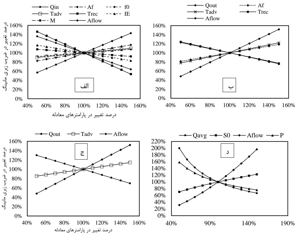
شکل ۲. آنالیز حساسیت پارامترهای ورودی معادله و درصد تغییر در ضریب زبری مانینگ. الف) ضریب زبری مانینگ در فاز پیشروی، ب) ضریب زبری مانینگ در فاز ذخیره، ج) ضریب زبری مانینگ در کل رخدادهای آبیاری و د) ضریب زبری مانینگ معادله.
