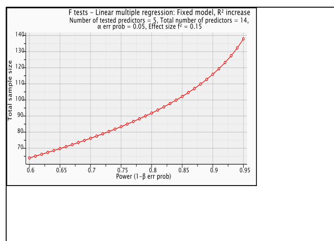
شکل ۳. برآورد حجم نمونه در نرم افزار G*Power
