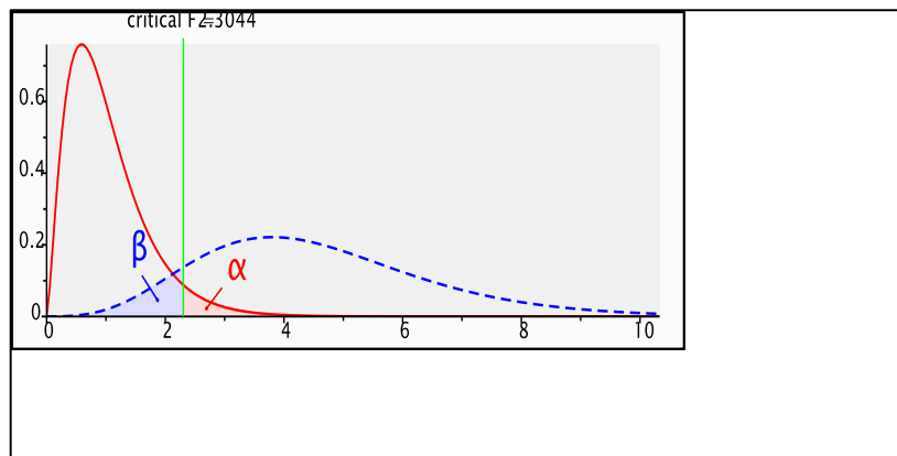
شکل ۲. برآورد حجم نمونه در نرم افزار G*Power
